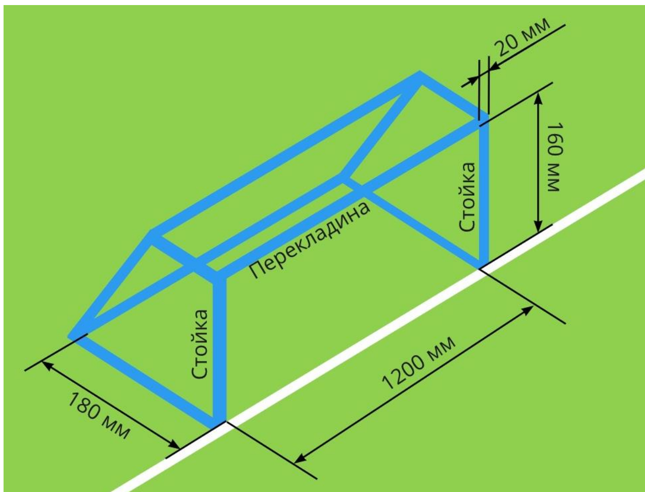
Рис. 6. Схема ворот
